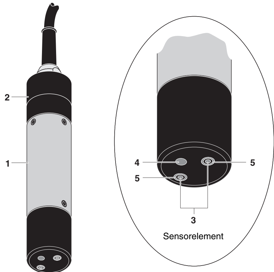
Bild 1-1 Aufbau der Leitfähigkeitsmesszelle TetraCon 700
